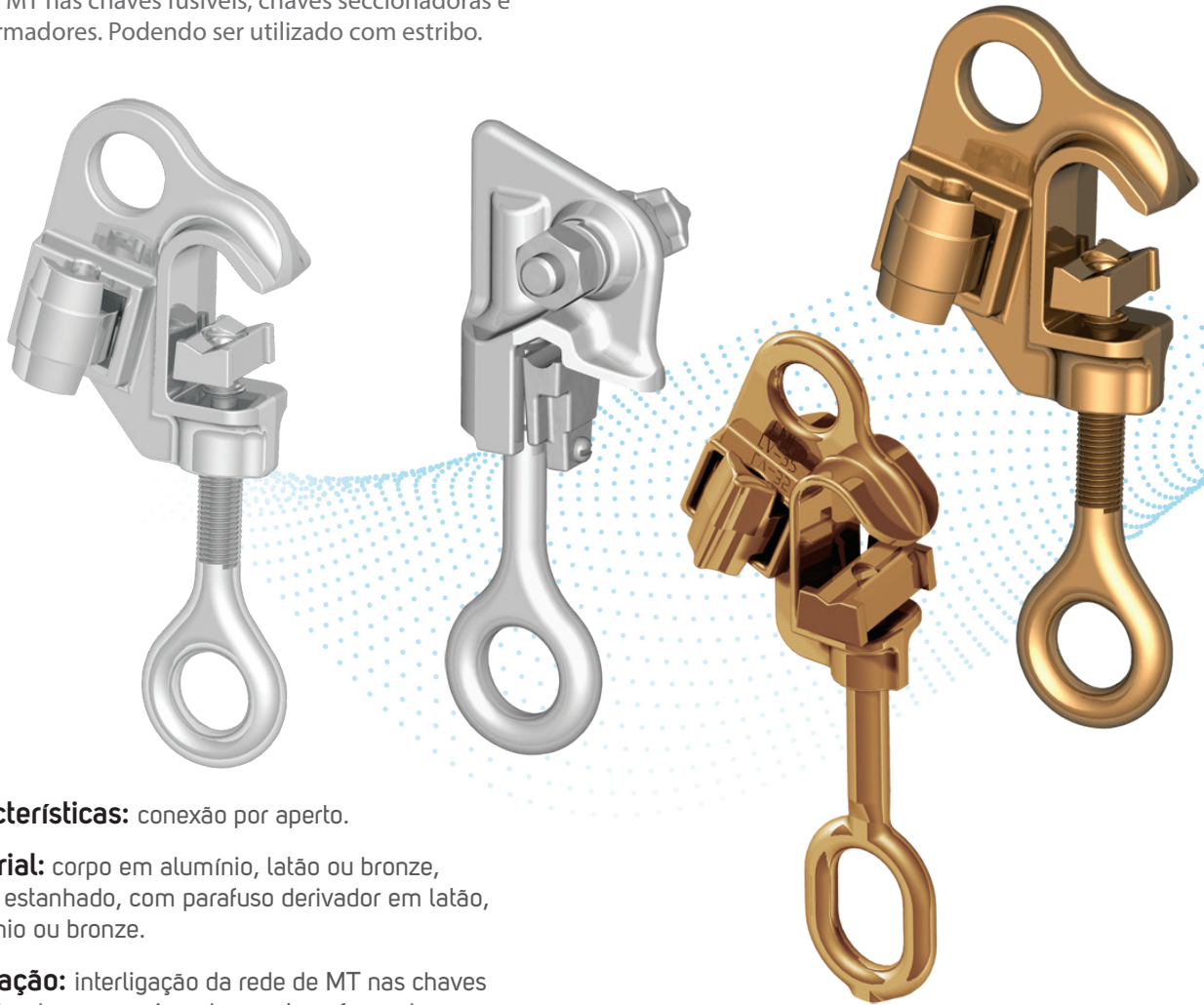
Grampo de Linha Viva
